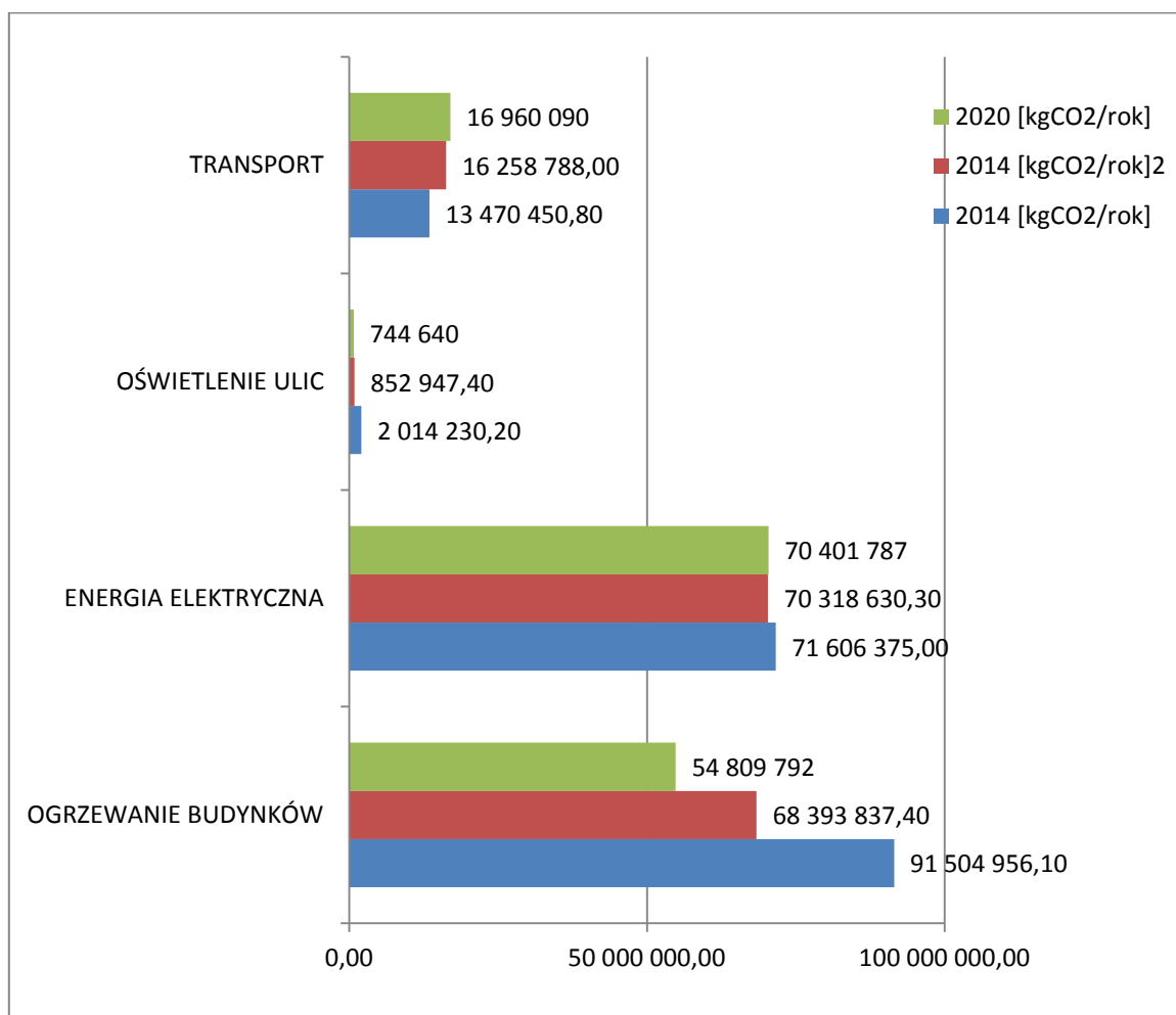
Rysunek 67. Porównanie źródeł emisji w gminie Bieruń w 1991, 2014 i 2020 roku.
