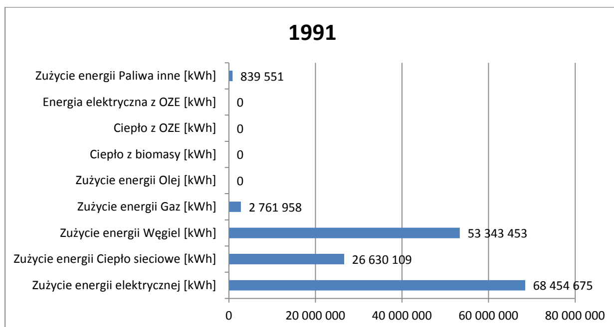
Rysunek 46. Struktura wykorzystania energii i paliw w 1991 roku w sektorze handel, usługi, przedsiębiorstwa.
