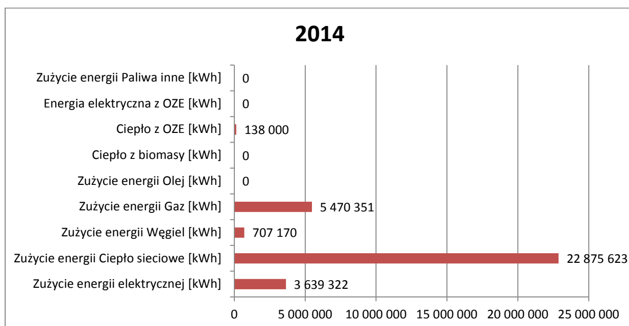
Rysunek 44. Struktura wykorzystania energii i paliw w 2014 roku w budynkach użyteczności publicznej.
