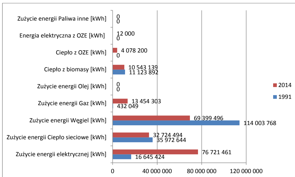
Rysunek 38. Porównanie struktury wykorzystania energii i paliw w 1991 i 2014 roku w budynkach mieszkalnych.
