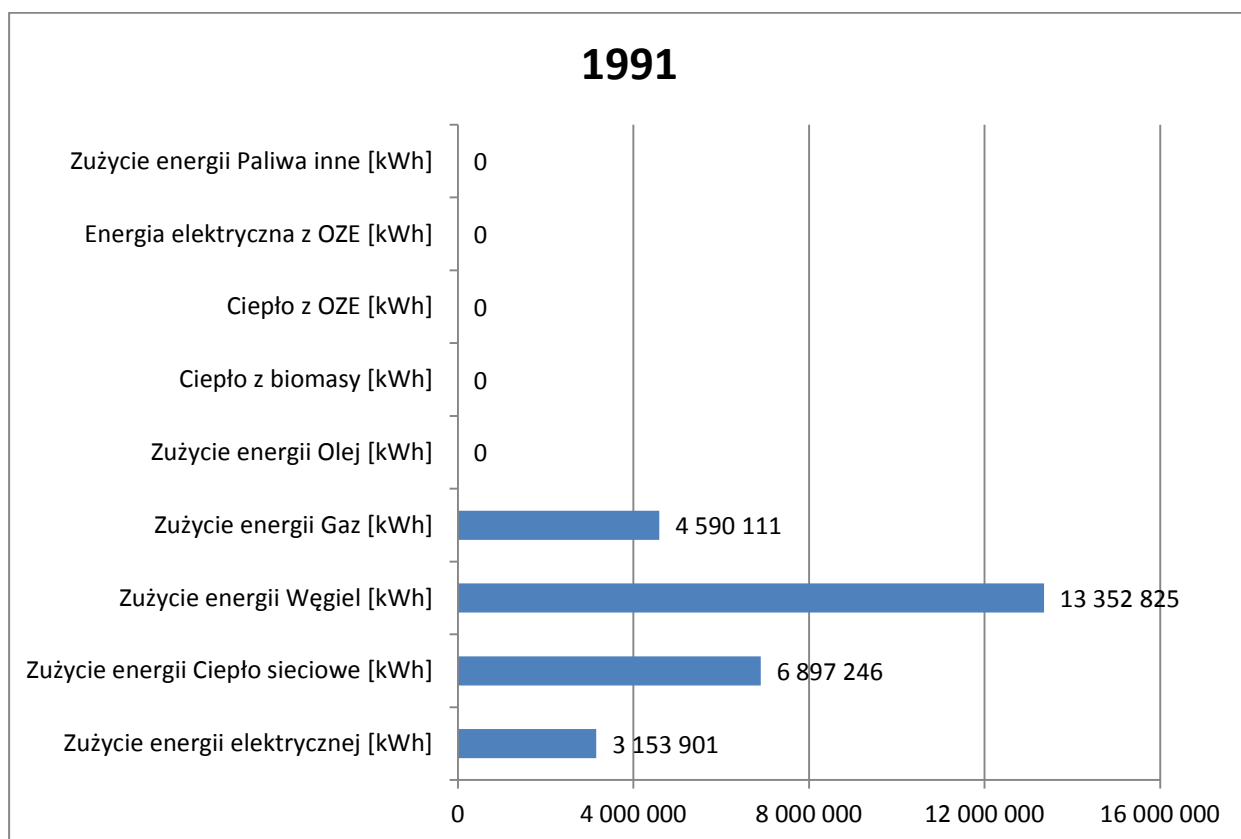
Rysunek 43. Struktura wykorzystania energii i paliw w 1991 roku w budynkach użyteczności publicznej.
