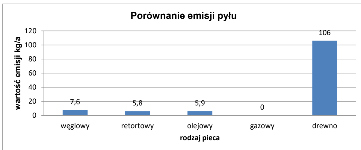
Rysunek 74. Porównanie emisji pyłu w zależności od rodzaju ogrzewania (pieca).
