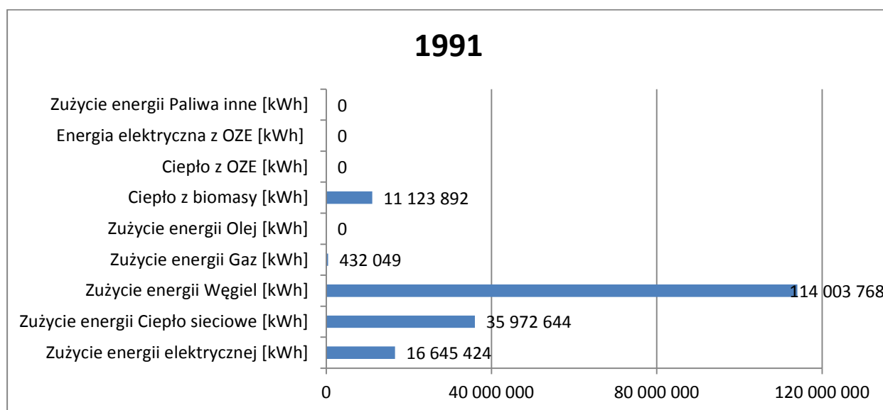
Rysunek 39. Struktura wykorzystania energii i paliw w 1991 roku w budynkach mieszkalnych.
