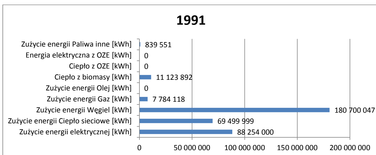
Rysunek 49. Porównanie struktury zużycia paliw w sektorze budynki w roku 1991.
