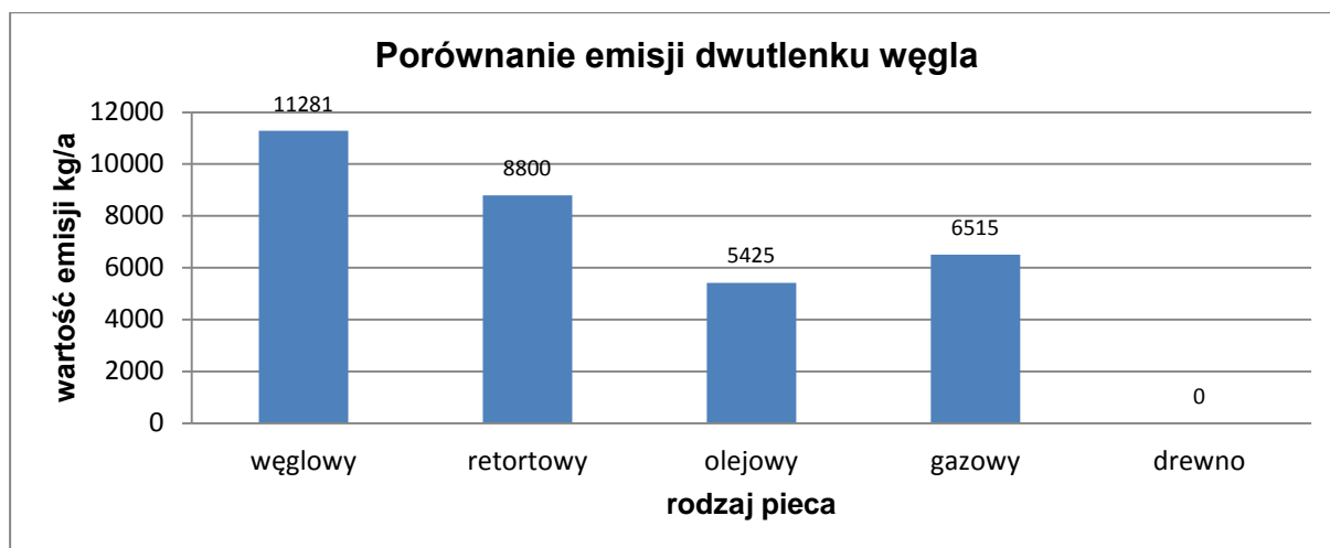
Rysunek 73. Porównanie emisji CO 2 w zależności od rodzaju ogrzewania (pieca).
