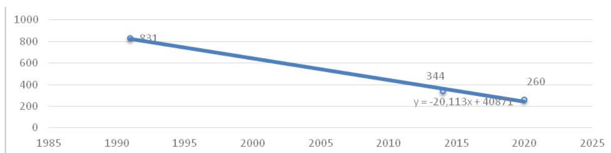
Rysunek 60. Emisja CO 2 pochodząca ze zużycia paliw do oświetlenia ulicznego w przeliczeniu na liczbę punktów świetlnych.
