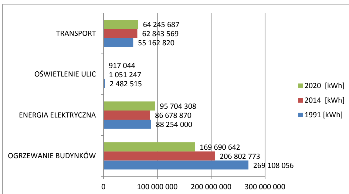
Rysunek 63. Porównanie wykorzystania energii w gminie Bieruń w 1991, 2014 i 2020 roku.
