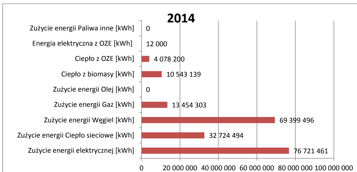
Rysunek 40. Struktura wykorzystania energii i paliw w 2014 roku w budynkach mieszkalnych.
