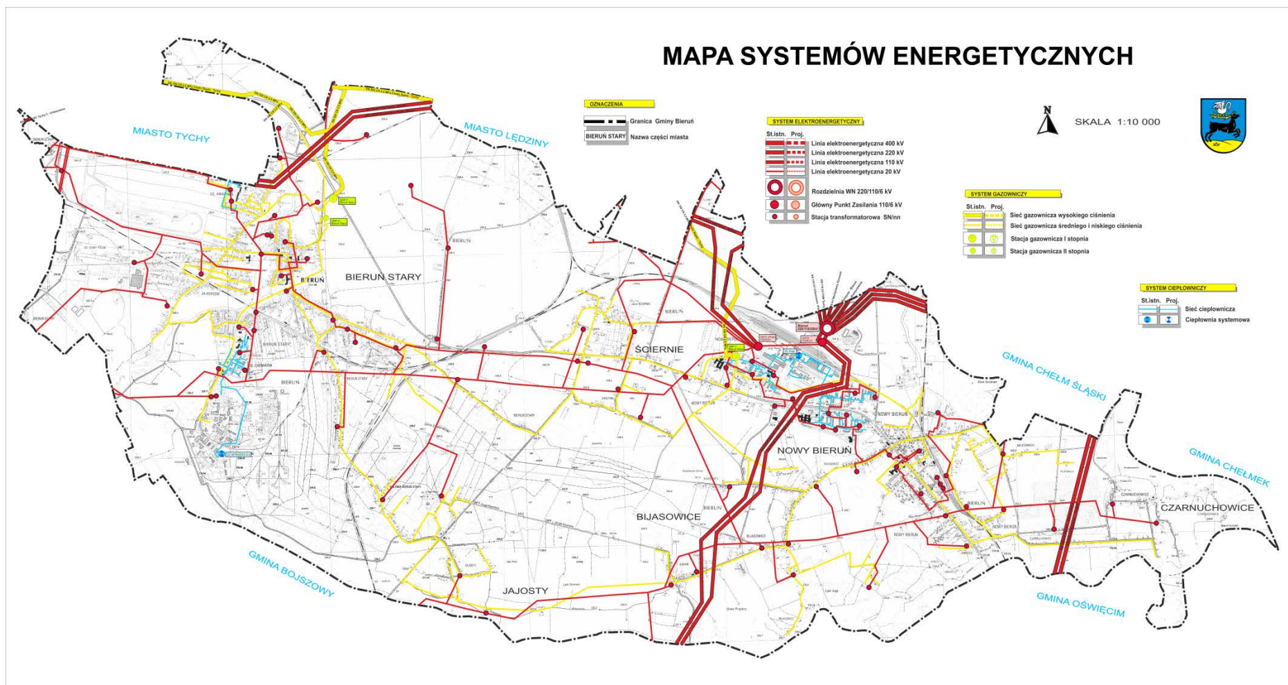
Rysunek 37. Mapa systemów energetycznych w gminie Bieruń (źródło: Projekt założeń do planu zaopatrzenia w ciepło, energię elektryczną i paliwa gazowe dla gminy Bieruń)
