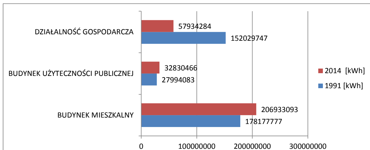
Rysunek 52. Porównanie struktury zużycia energii wg sektorów w roku 1991 i 2014.
