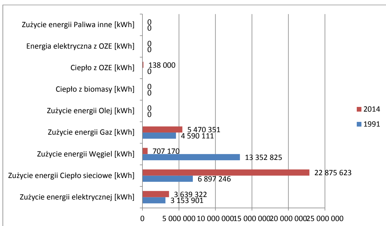
Rysunek 42. Porównanie struktury wykorzystania energii i paliw w 1991 i 2014 roku w budynkach użyteczności publicznej.
