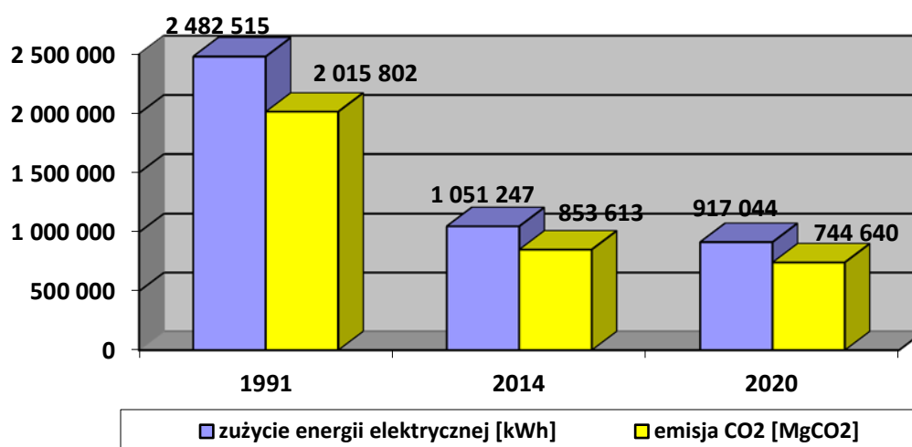
Rysunek 59. Prognozowane zmiany w zużyciu i emisji energii elektrycznej niezbędnej do zapewnienia oświetlenia ulicznego w gminie Bieruń w 1991, 2014 i 2020 roku.
