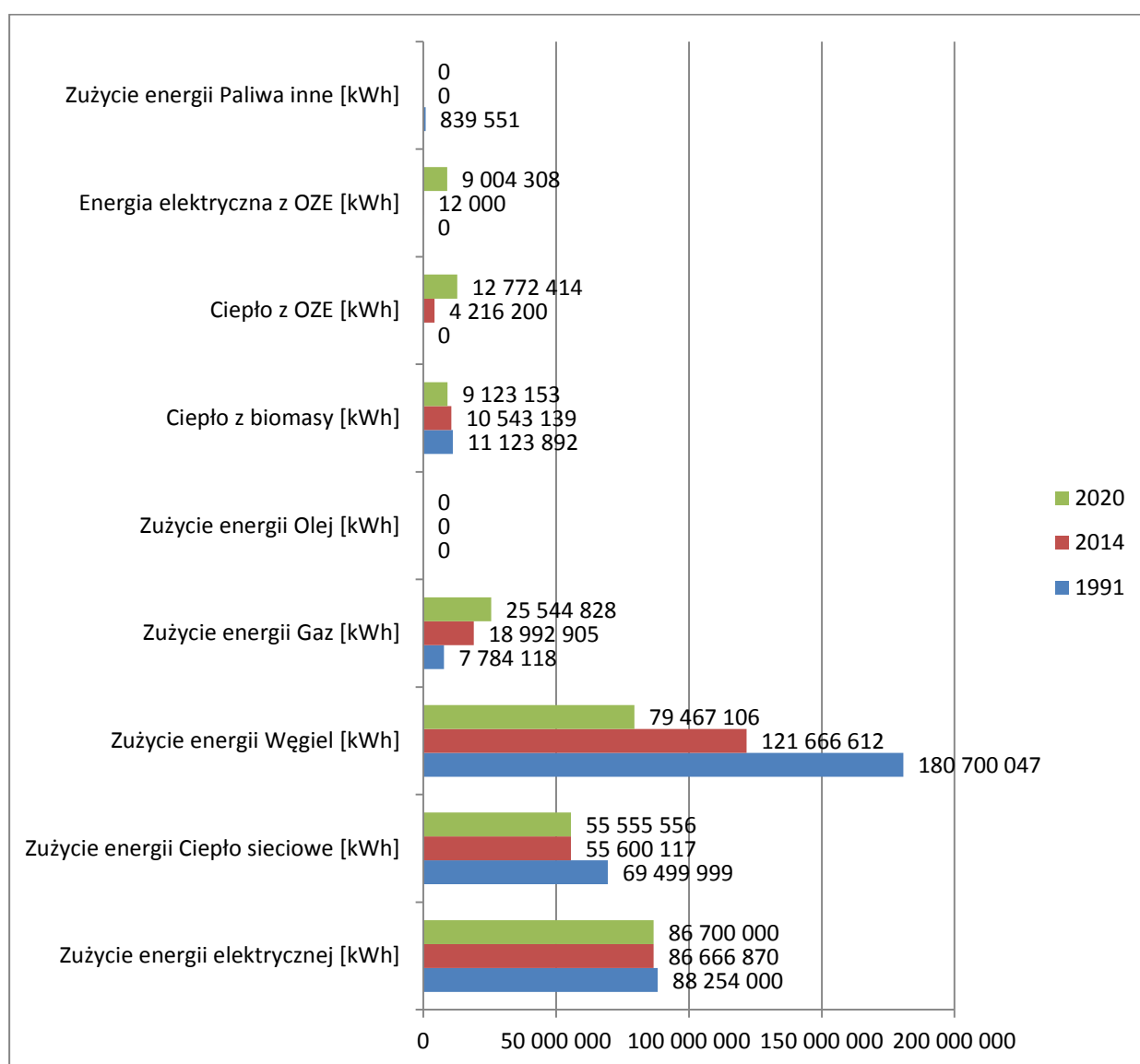
Rysunek 48. Struktura zużycia energii dla sektora budynki (1991, 2014 i 2020 rok).
