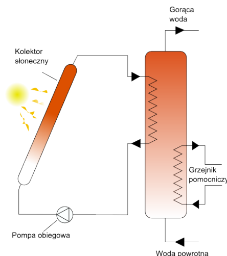
Rysunek 76. Uproszczony schemat działania kolektora słonecznego (źródło: http://ogrzewanie.drewnozamiastbenzyny.pl/kolektor-sloneczny/ ).
