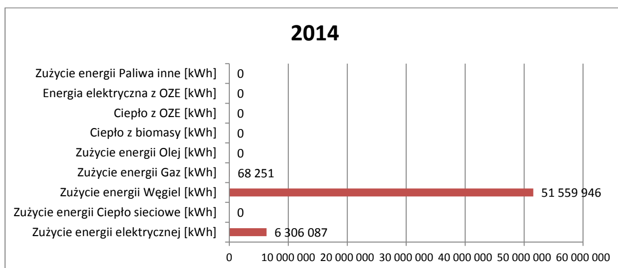
Rysunek 47. Struktura wykorzystania energii i paliw w 2014 roku w sektorze handel, usługi, przedsiębiorstwa.
