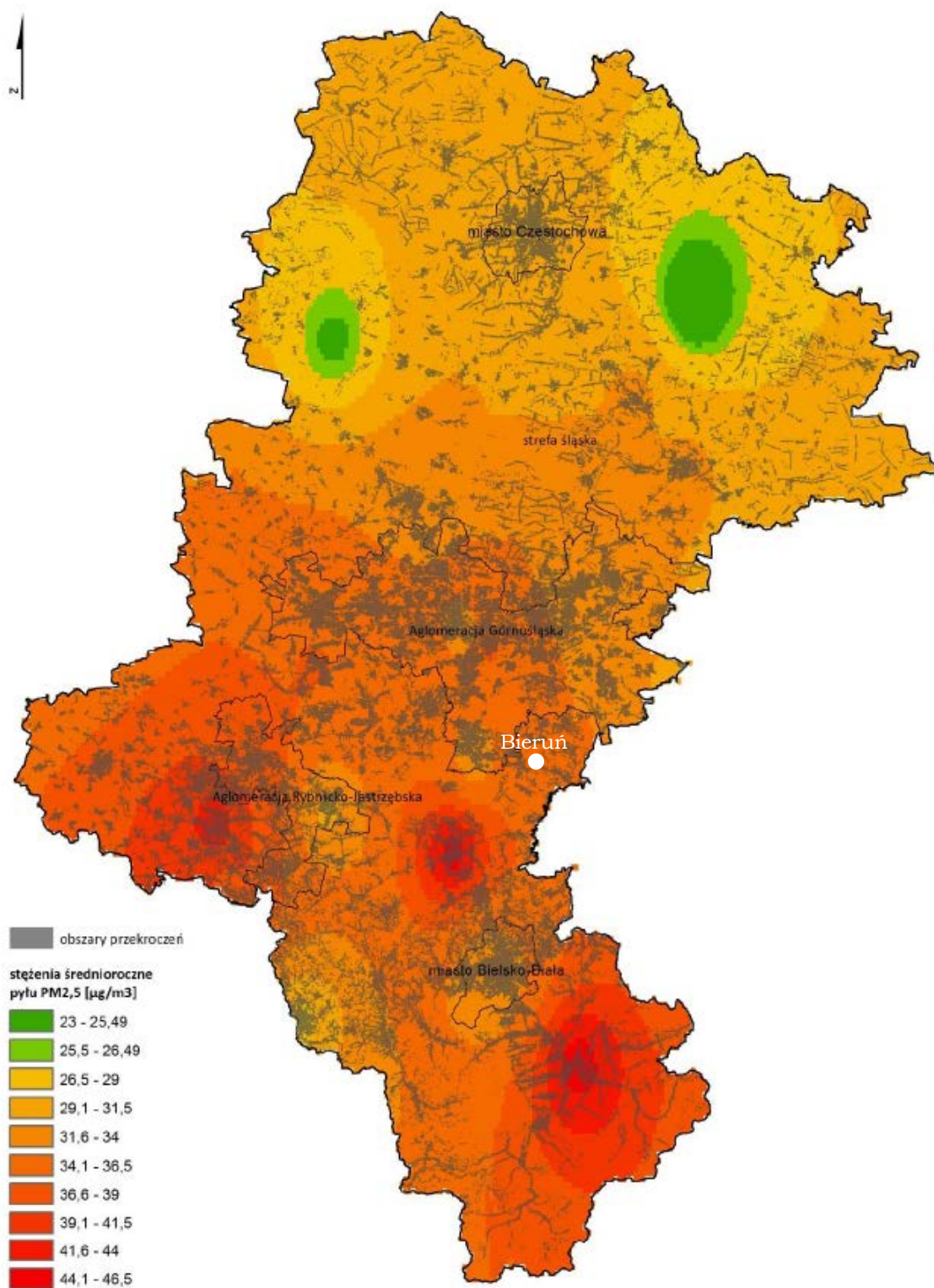
Rysunek 34. Obszary przekroczeń średnich stężeń rocznych pyłu PM 2.5 - kryterium ochrona zdrowia ludzi (źródło: Dwunasta roczna ocena jakości powietrza w województwie Śląskim, obejmująca 2013 rok)
